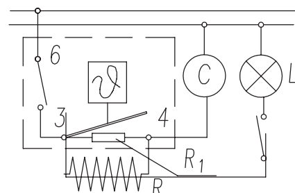
SCHEMA TIPICO DI COLLEGAMENTO typical wiring diagram
